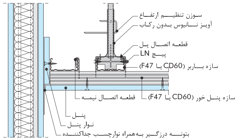
D-112-AW06 اتصال سقف کاذب دارای کد حریق به دیوار کی پلاس (لغزان)
