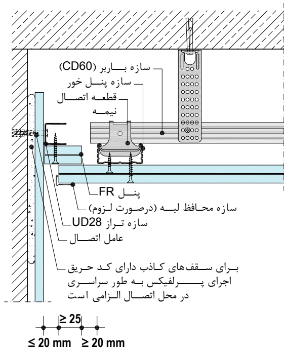
D-112-AW08 (دارای خط سایه) اتصال سقف کاذب دارای کد حریق به دیوار بنیایی
