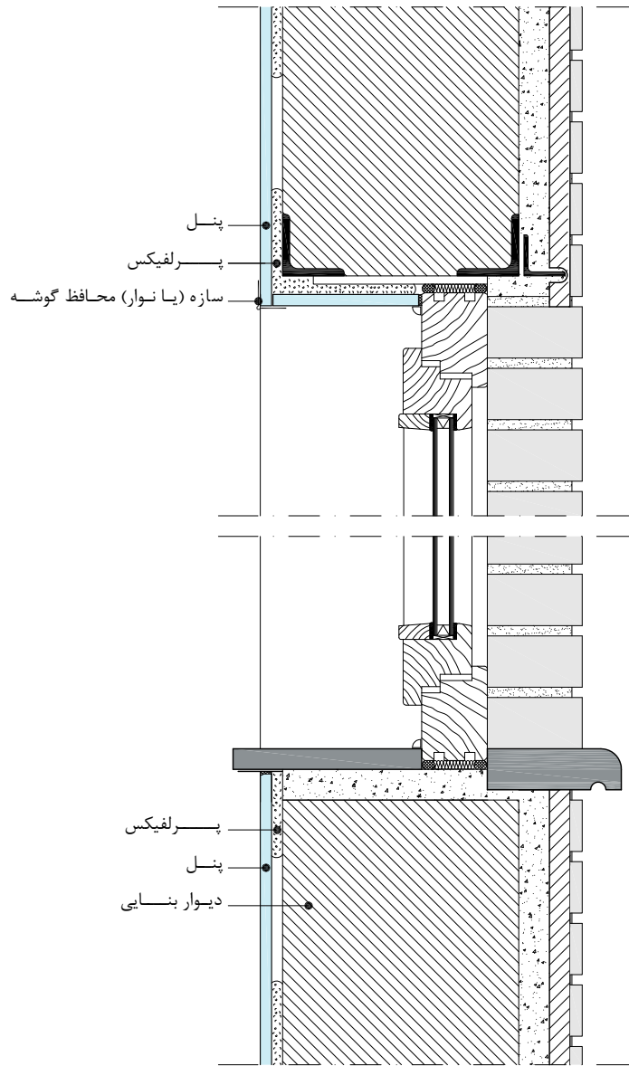
W611-001 پوشش کاری دور پنجره و جزئیات نصب سنگ کف پنجره
