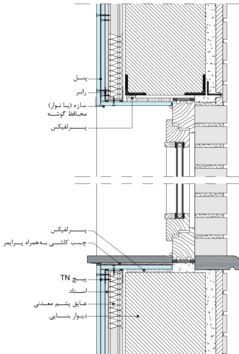
W626-001 پوشش کاری دور پنجره و جزئیات نصب سنگ کف پنجره
